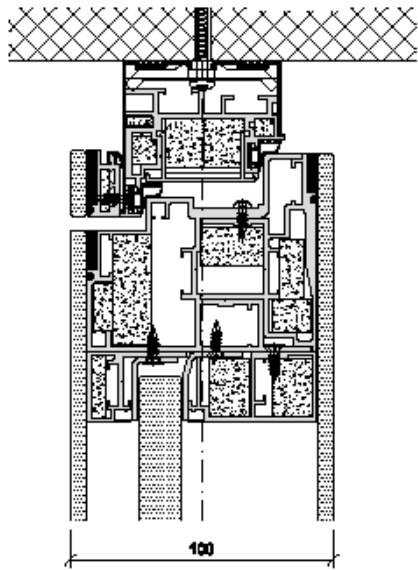
Vertikalschnitt
