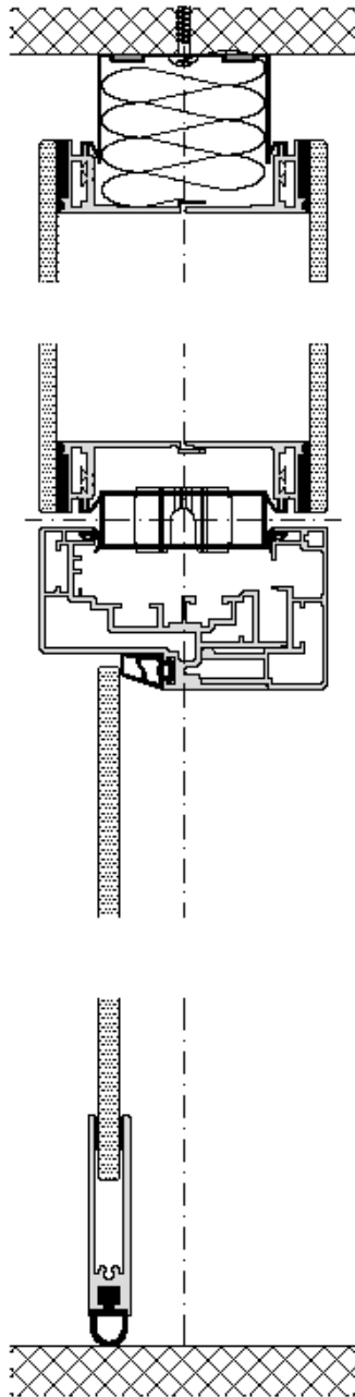
Vertikalschnitt
