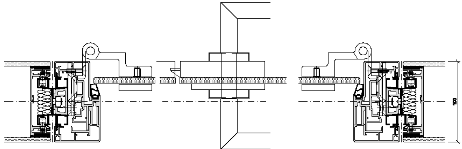
Horizontalschnitt
