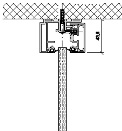
Deckenanschluss
