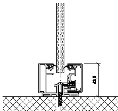
Bodenanschluss
