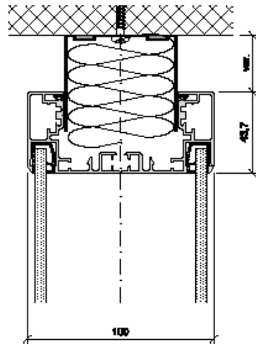
Deckenanschluss
