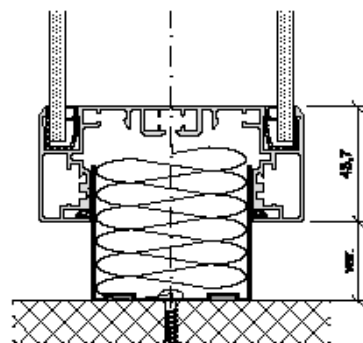
Bodenanschluss
