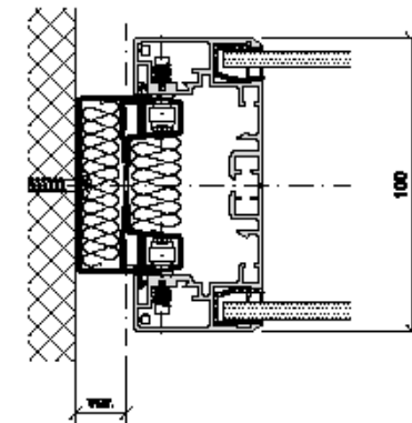
Anschluss variabel
