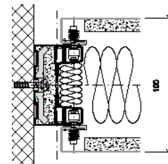
Anschluss variabel
