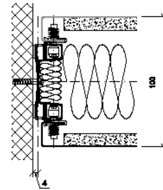
Wandanschluss
