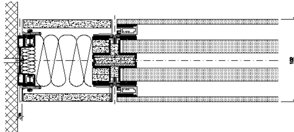
Wandanschluss
