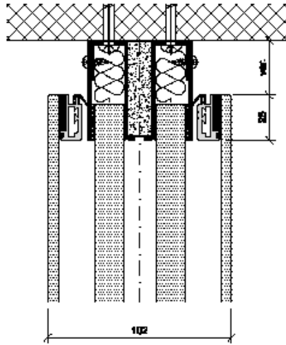
Deckenanschluss
