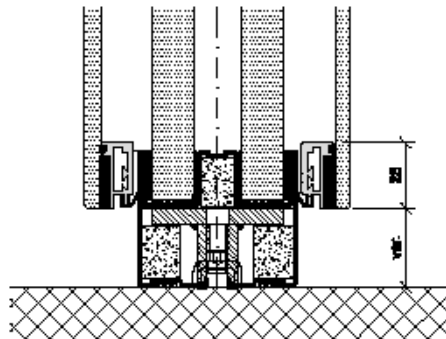
Bodenanschluss
